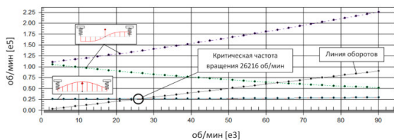
Рис. 5. Карта собственных частот роторной системы
