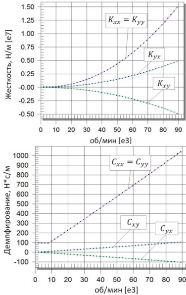
Рис. 4. Кривые коэффициентов жесткости и демпфирования
