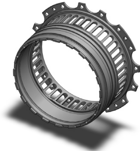
Рис. 1. «Беличье колесо» с прямыми стержнями с прямоугольным сечением
