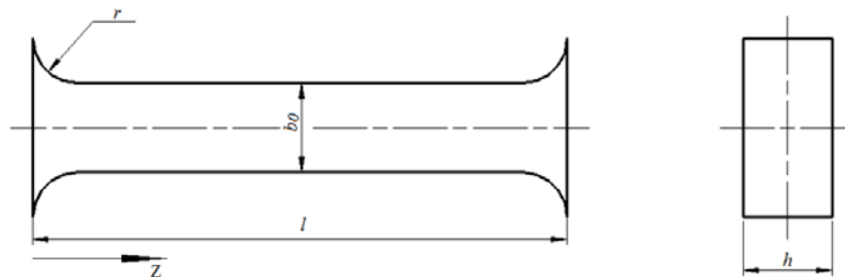
Рис. 2. Конструкция стержневого элемента «беличьего колеса»: h – высота, b_0 – ширина в центральной части, r – радиус скругления пазов, l – длина
