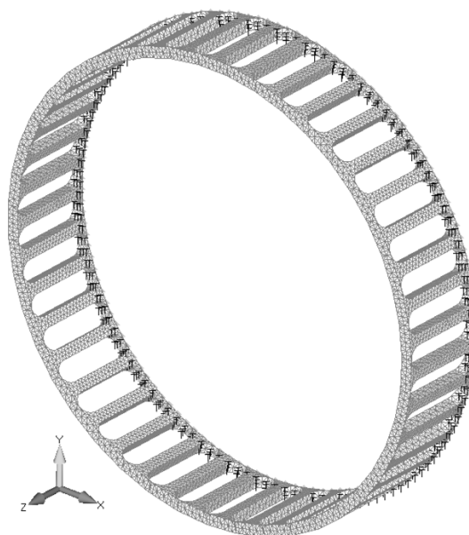
Рис. 3 Конечно-элементная модель стержневых элементов «беличьего колеса»
